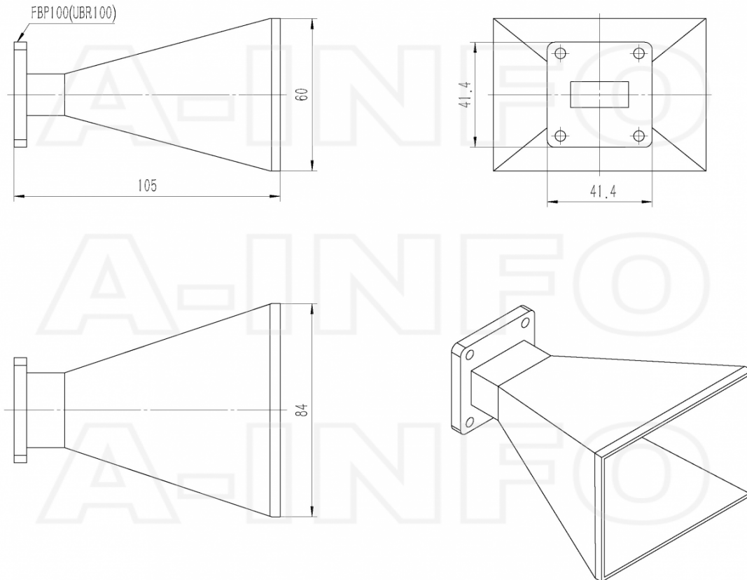
FBP100 Output (P/N: LB-90-15-A)
